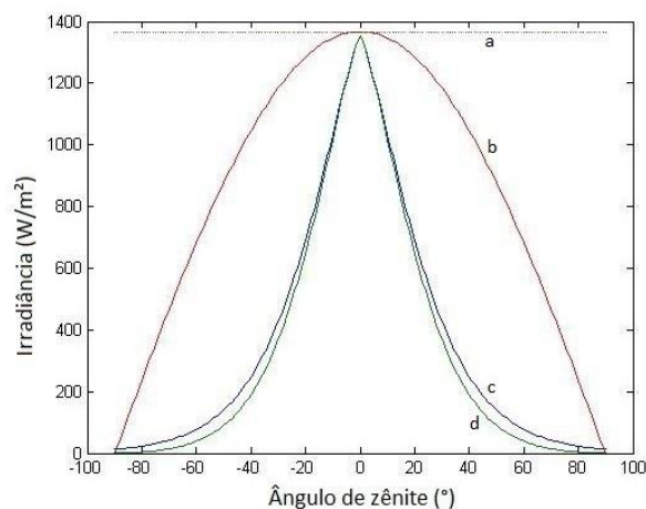
Figura 2 – Curvas de irradiância de acordo com atenuância atmosférica pelo método de Vianello e Alves (1991)
