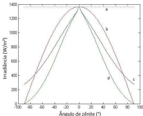
Figura 3 - Curvas de irradiância de acordo com atenuação atmosférica pelo método de Janjai (2010)
